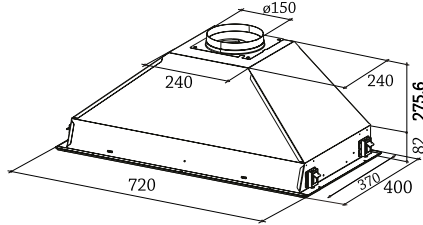
INBOUW AFZUIGKAP
