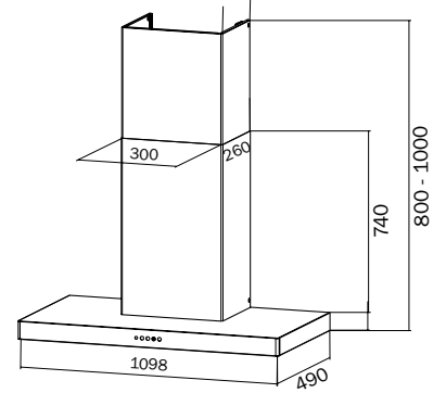
FLAT AFZUIGKAP
