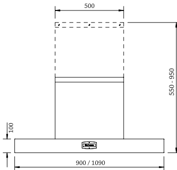
MODERNE AFZUIGKAP
